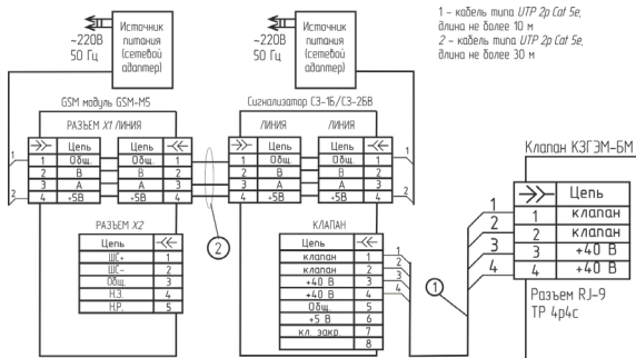
Рис. А2. Схема электрических соединений сигнализаторов C3-хБ, электромагнитного клапана КЗГЭМ-БМ и GSM модуля CGK GSM-M5.
