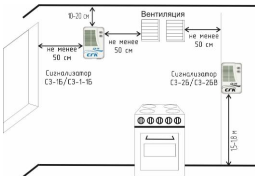
Рис.2 Схема размещения сигнализаторов загазованности СЗ-Б.
