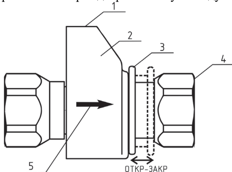
Рисунок 2. – Клапан КЗГЭМ-БМ.
