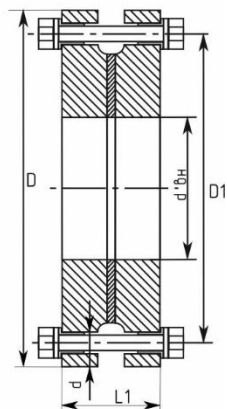
Рисунок 3 - Изолирующее фланцевое соединение ИФС-В
