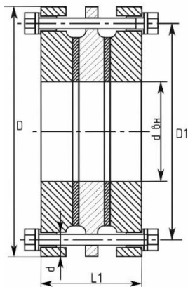
Рисунок 2 - Изолирующее фланцевое соединение ИФС-Б
