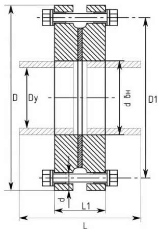
Рисунок 1 - Изолирующее фланцевое соединение ИФС-А
