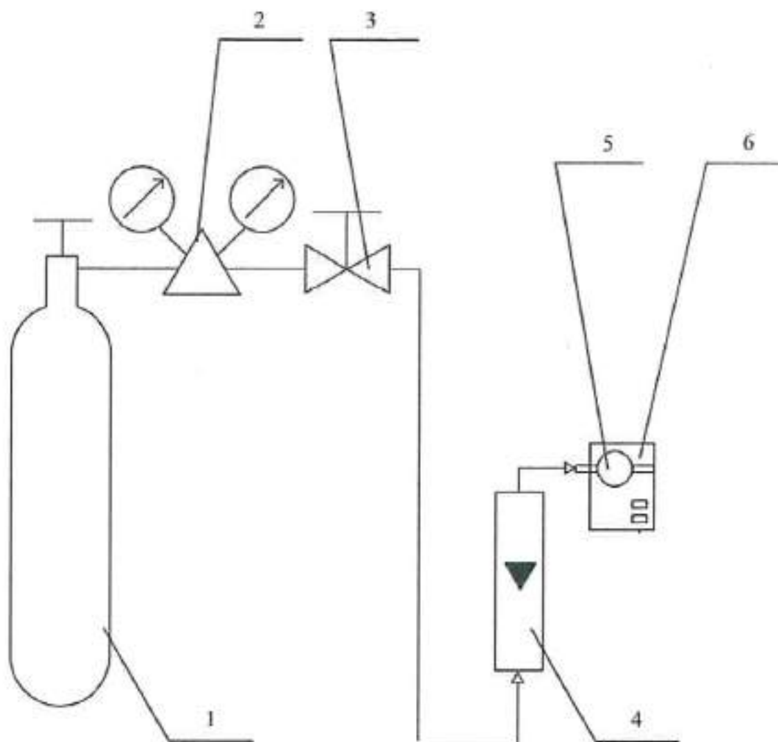
Рисунок Б.1 – Рекомендуемая схема подачи ГС на вход сигнализаторов загазованности бытовых СЗ-Б
