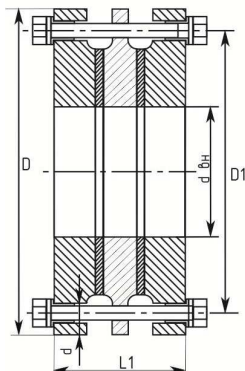
Рисунок 3 - Изолирующее фланцевое соединение ИФС-Б
