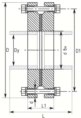
Рисунок 2 - Изолирующее фланцевое соединение ИФС-А
