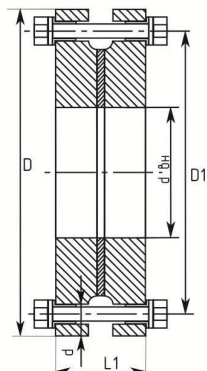
Рисунок 4 - Изолирующее фланцевое соединение ИФС-В
