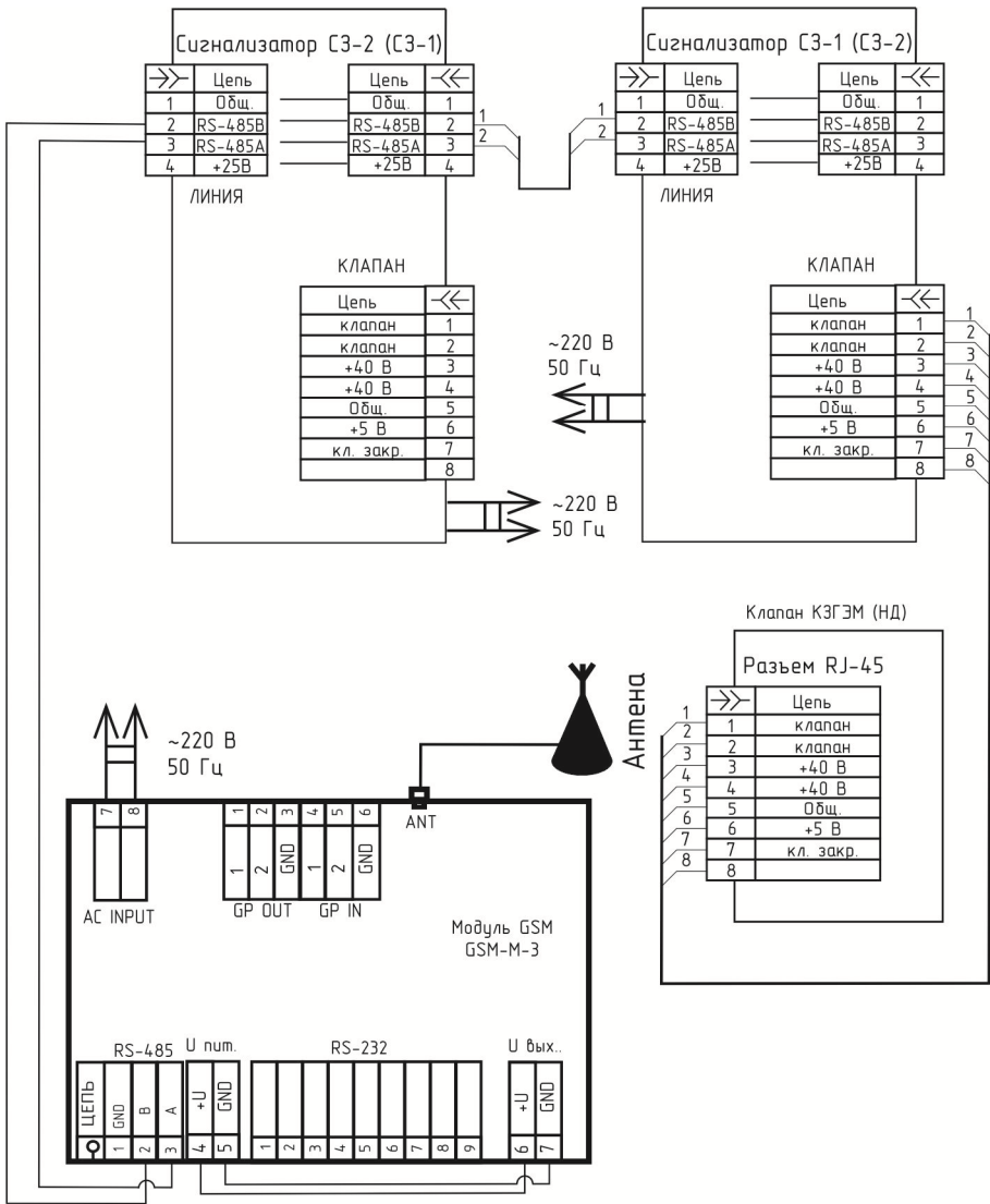
Рис 2. Схема подключения изделия к системе автономного контроля Загазованности СГК-2
