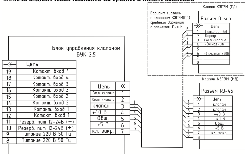
Рис 1. Схема подключения КЗГЭМ (НД) с разъемом RJ-45 и КЗКЭМ (СД) с разъемом D-sub.
